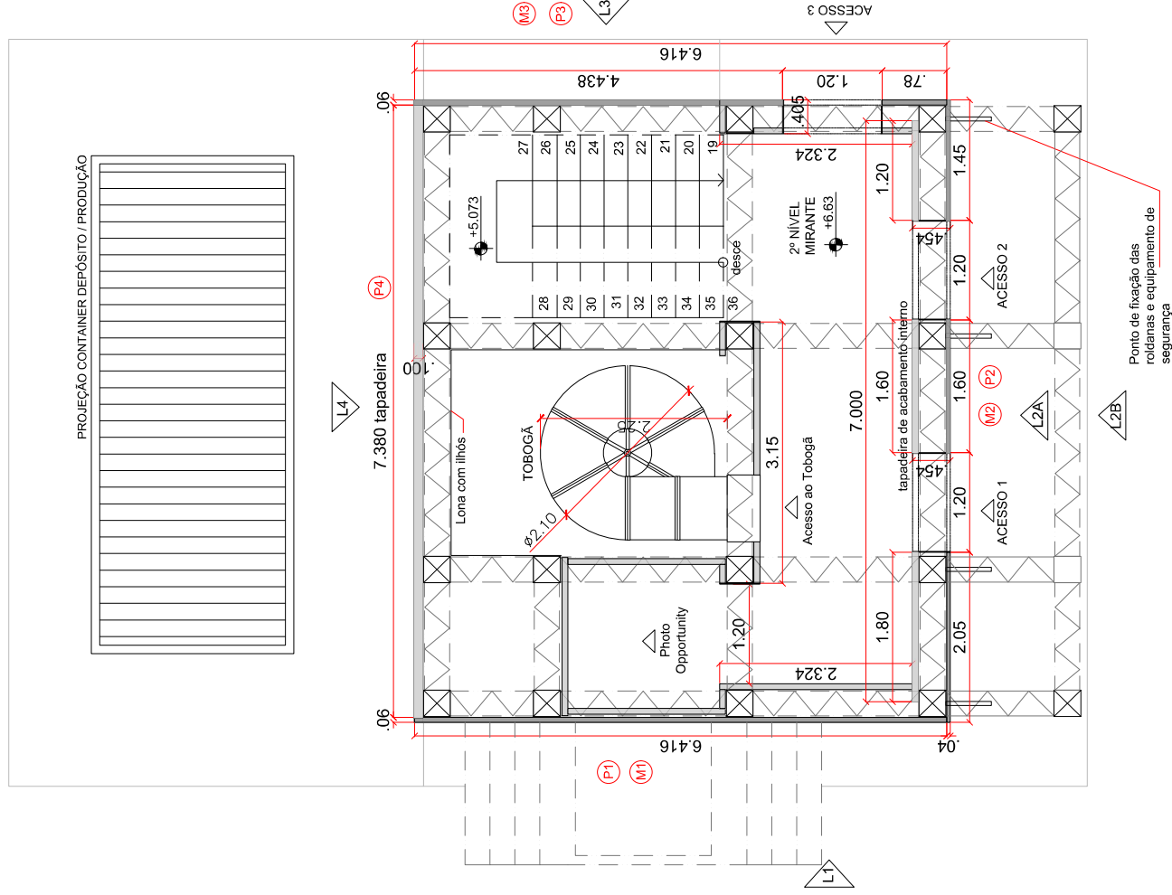
PLANTA BAIXA - 2º NÍVEL / MIRANTE
